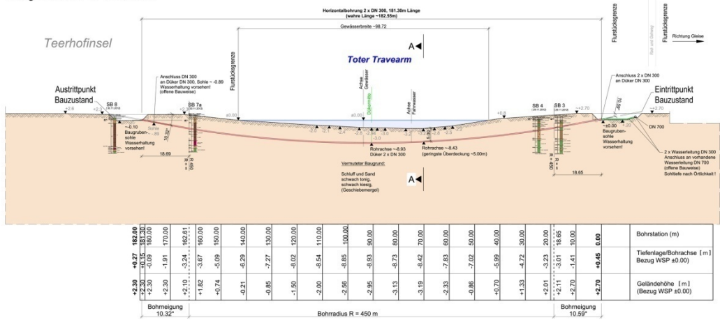
Längsschnitt B-B M. 1 : 500
